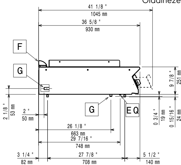
Oldalnézet
